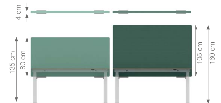
Ausführung Höhe 2 (links) und Höhe 1 (rechts) Variant height 2 (left) and height 1 (right)
